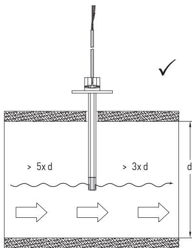
Schéma de montage
