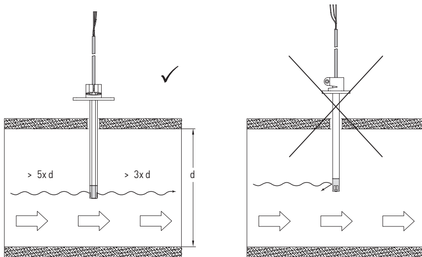
Схема монтажа
